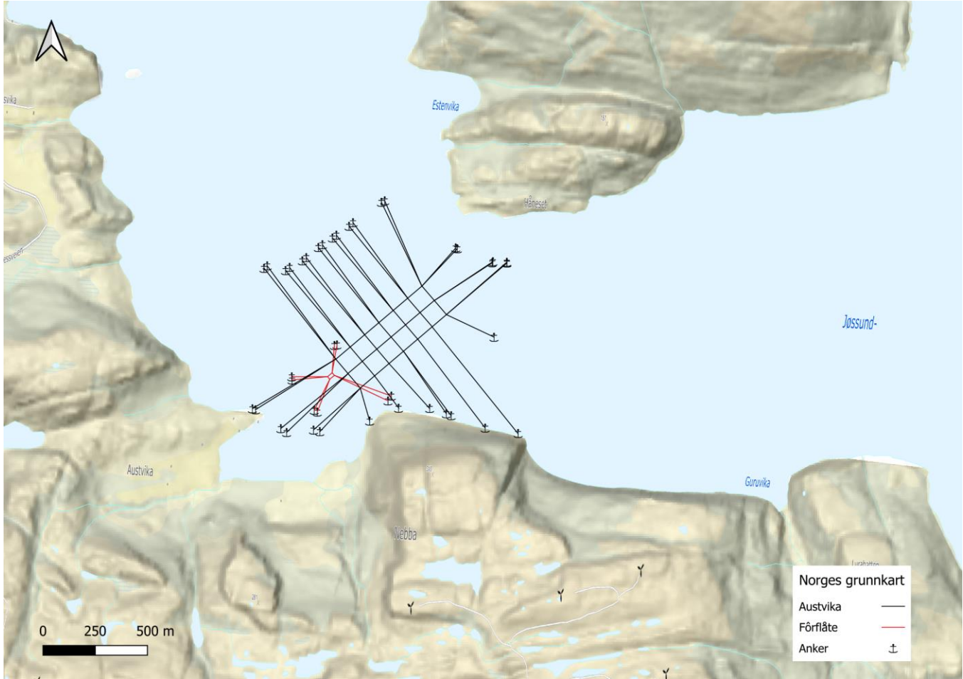
Figur 1: Anleggsskisse
